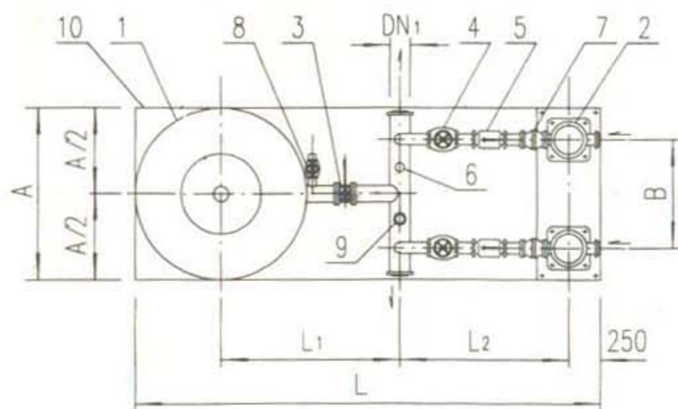
平面图
