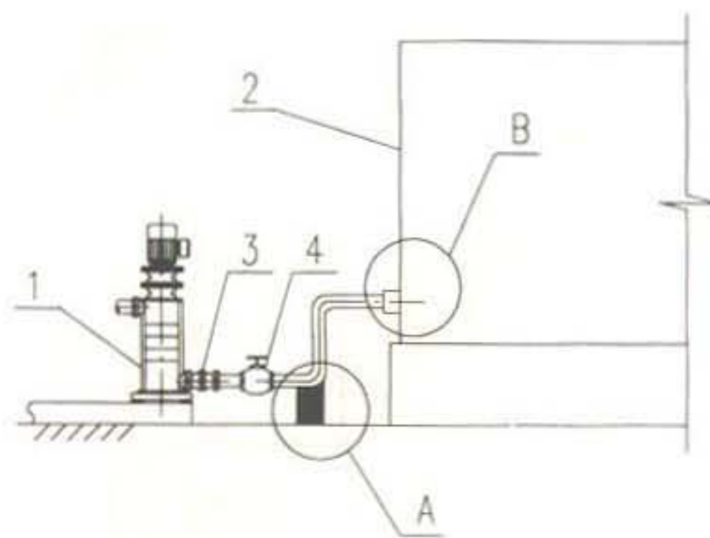
水泵吸水管安装
