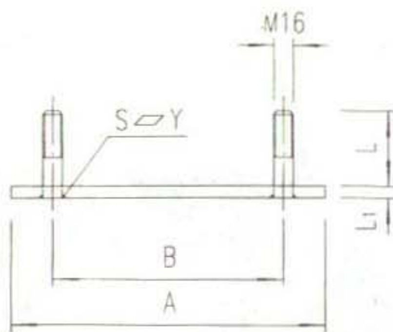
钢垫板立面图
