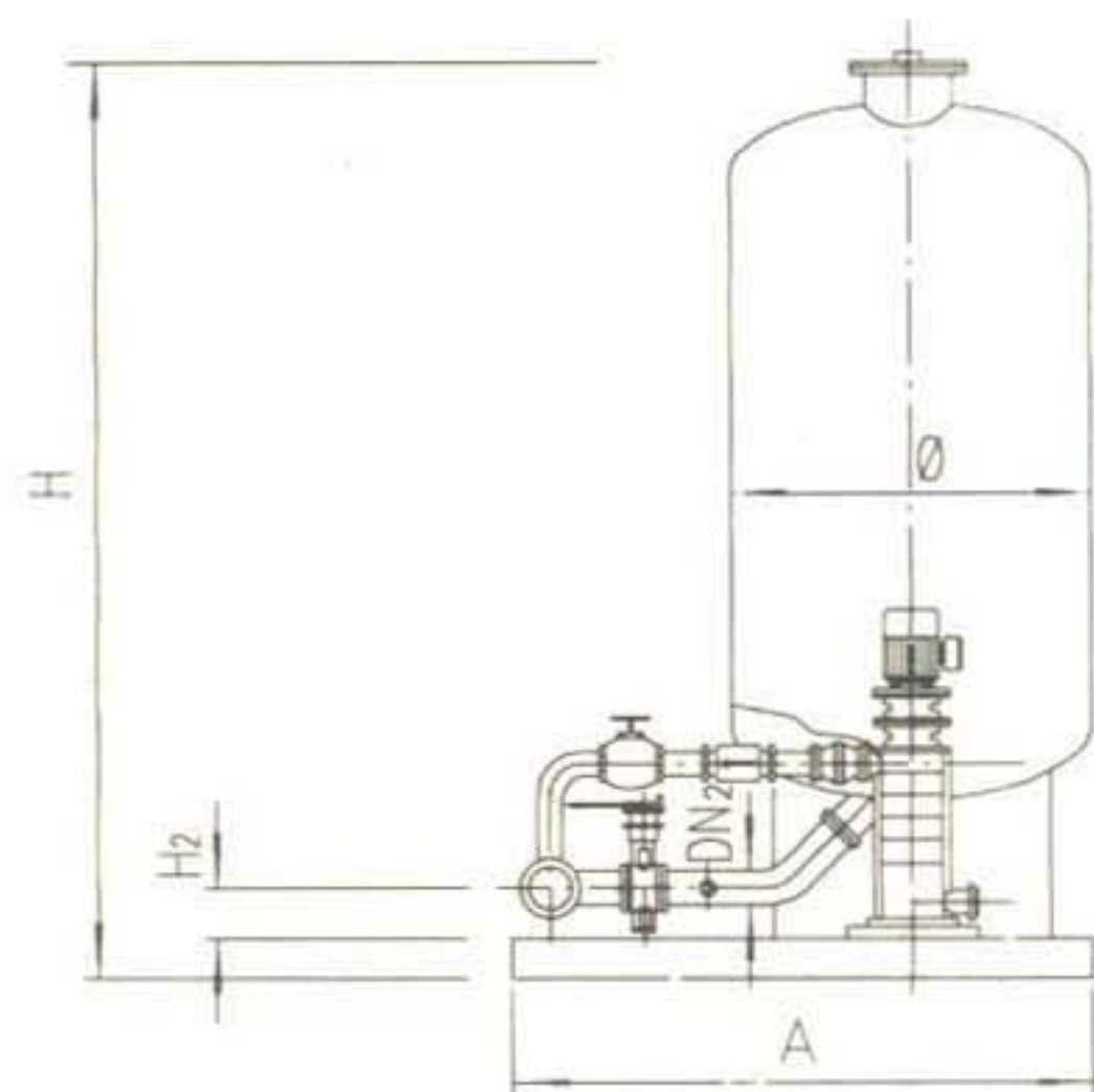
右立视图
