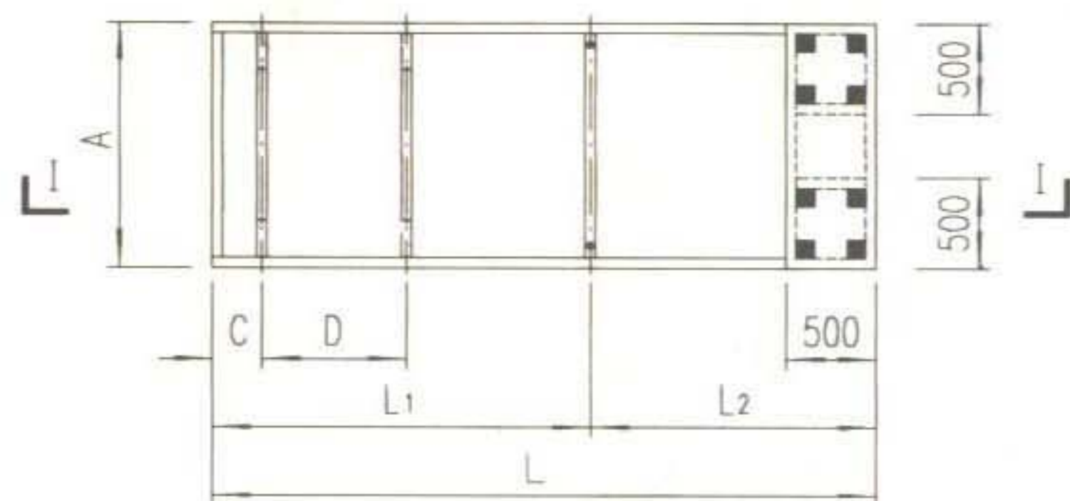
甲型底座平面
