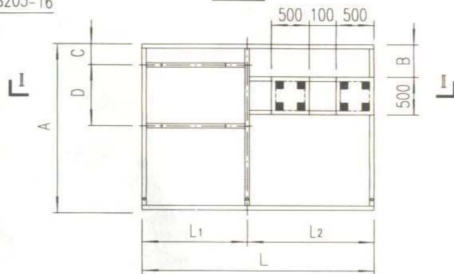
乙型底座平面
