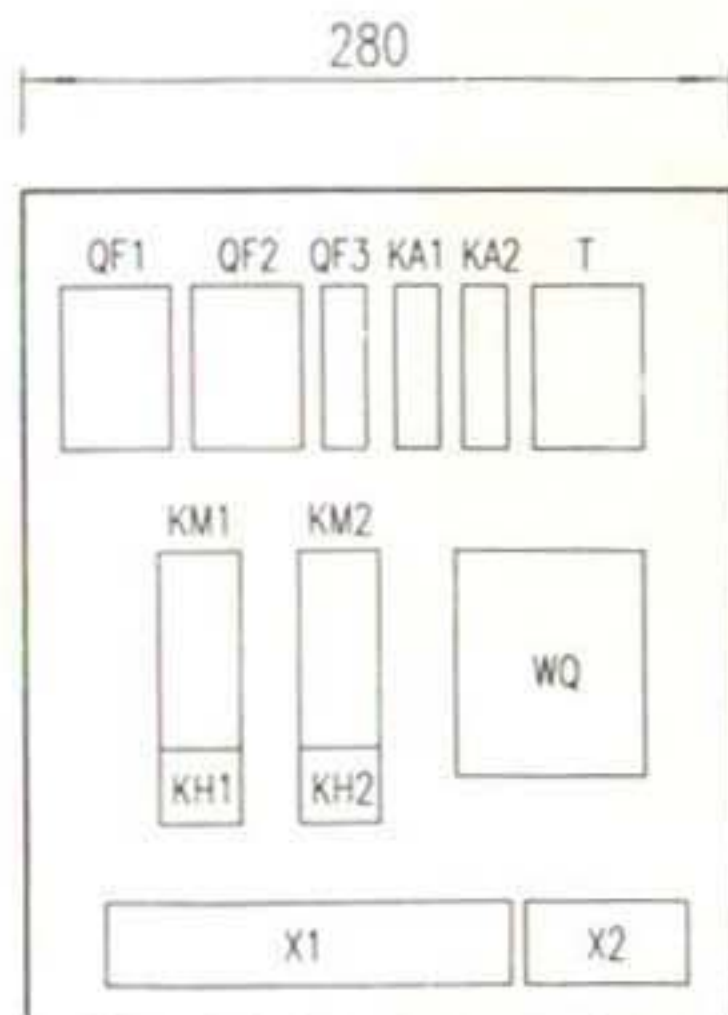
箱内元件布置图
