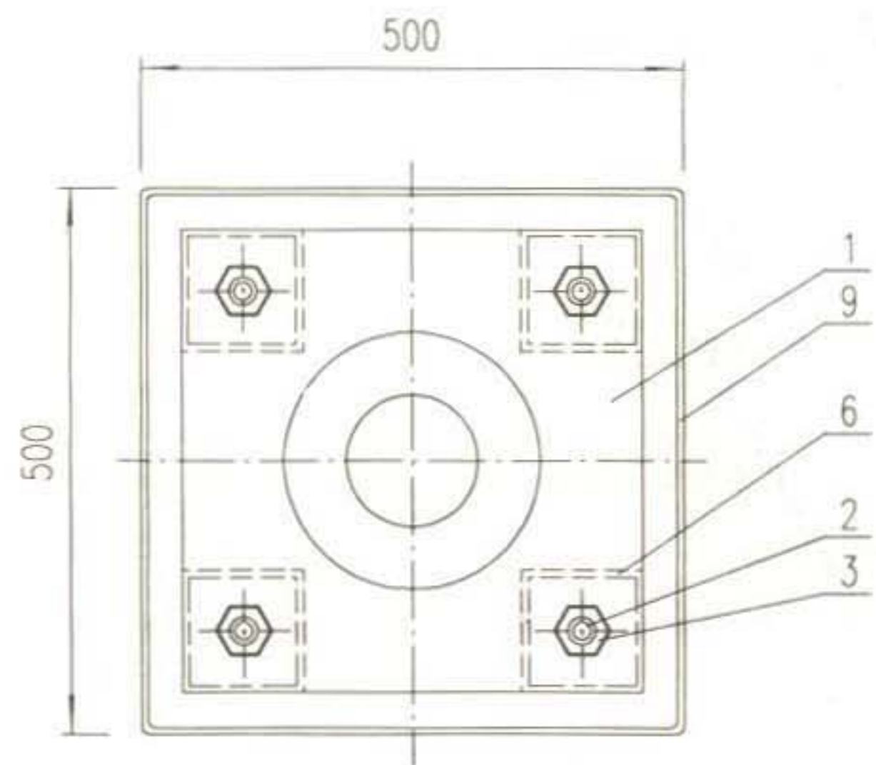
平面图
