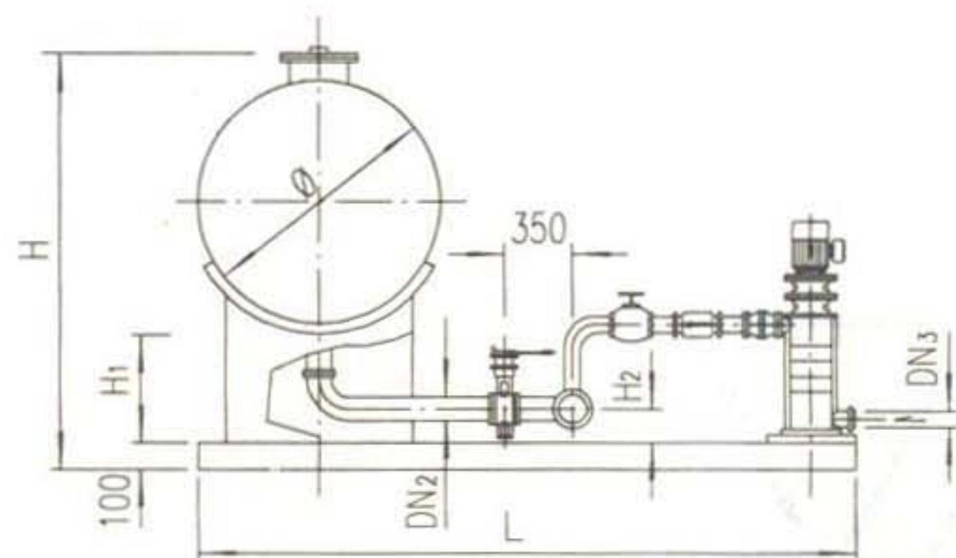
立视图
