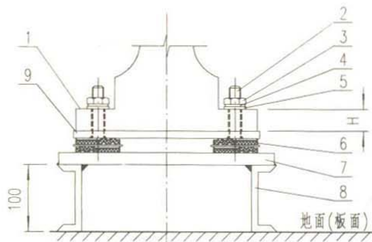
立面图
