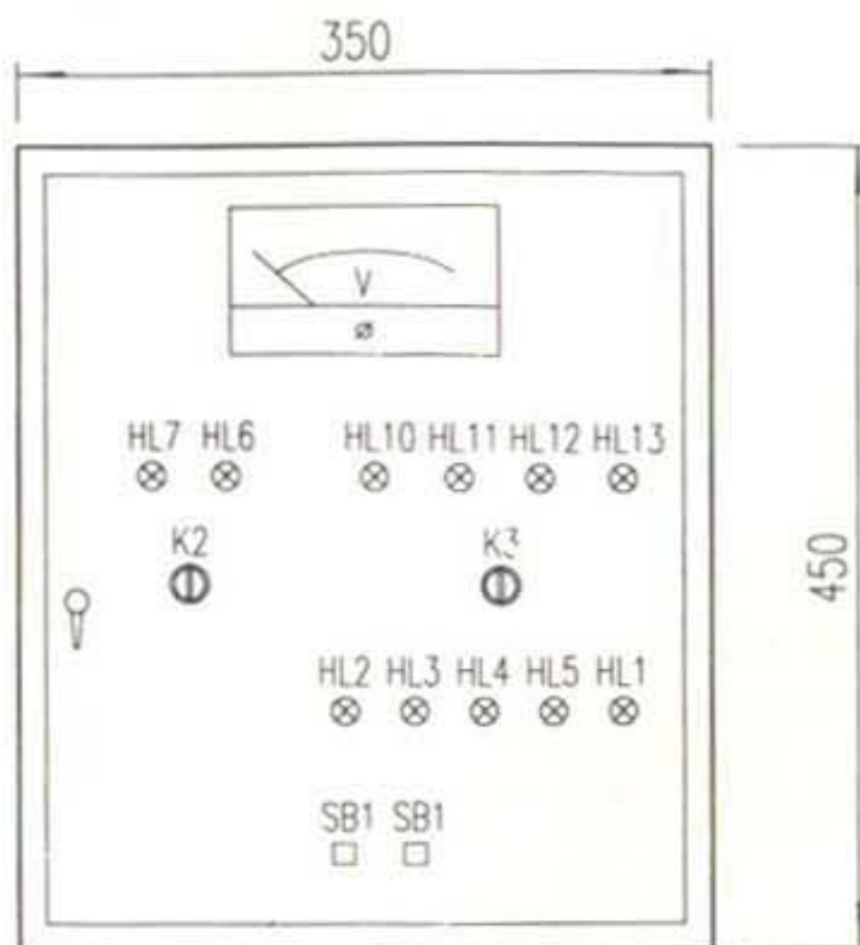
箱面元件布置图
