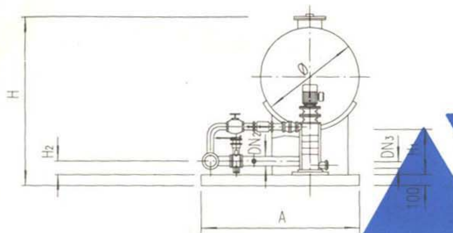
右立视图
