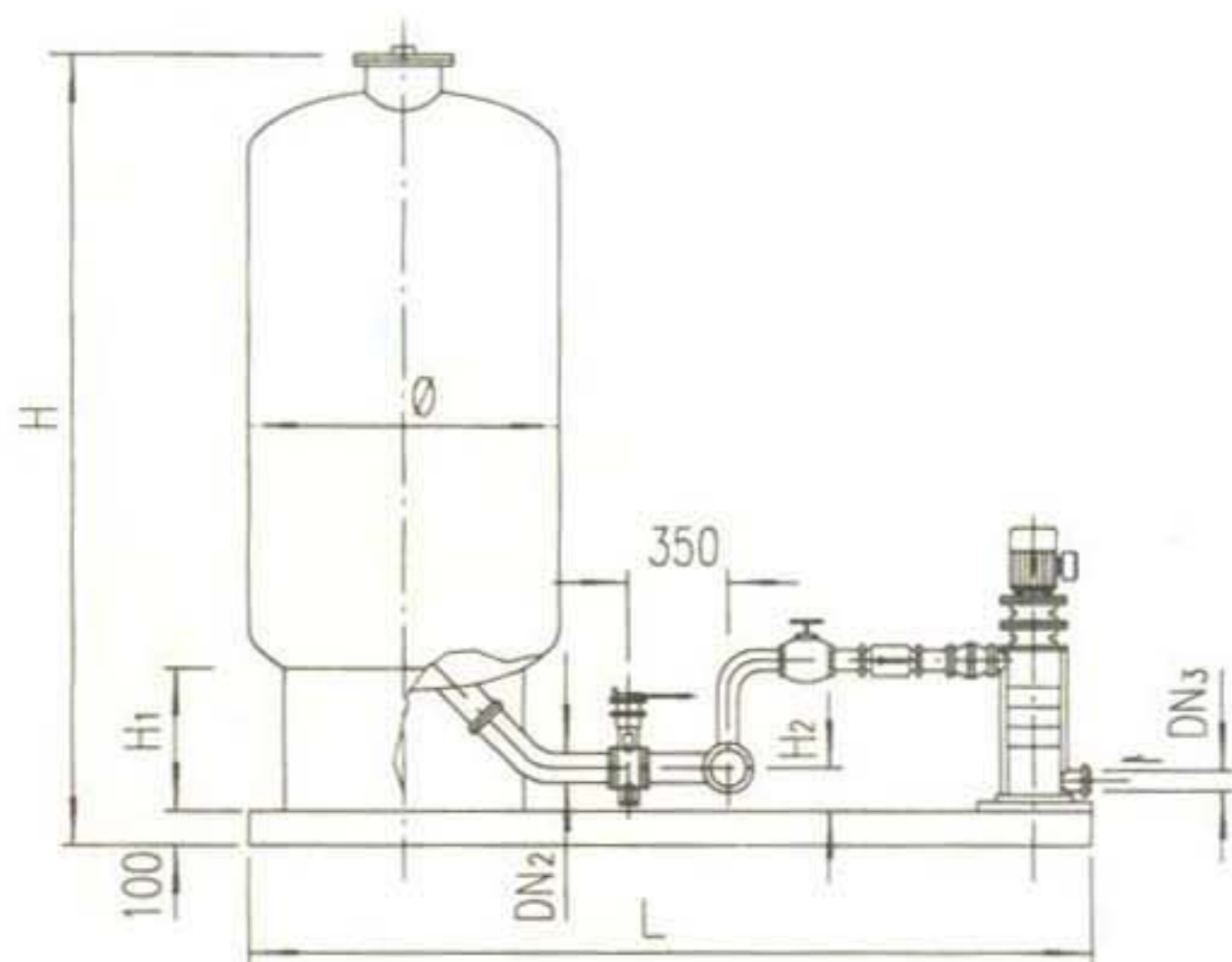
立视图
